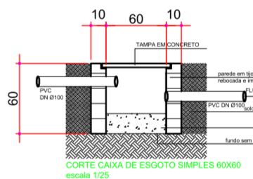
CORTE CAIXA DE ESGOTO SIMPLIS 60X60 escala 1/25
