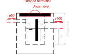
Caixa de gordura Corte 1 - ESC. 1:25
