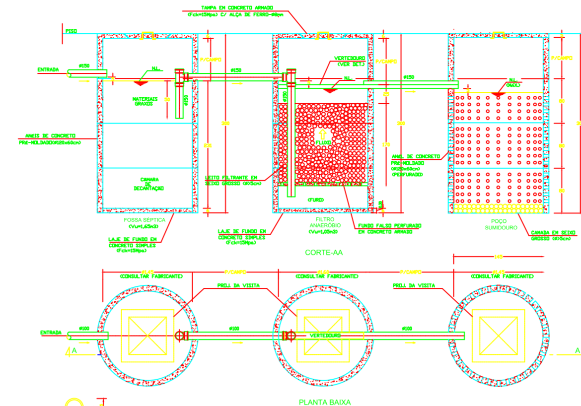
DETALHE DO VERTEDOURO ESC. 1/10 DETALHE- (SISTEMA DE TRATAMENTO DE ESGOTO) ESC. 1/25
